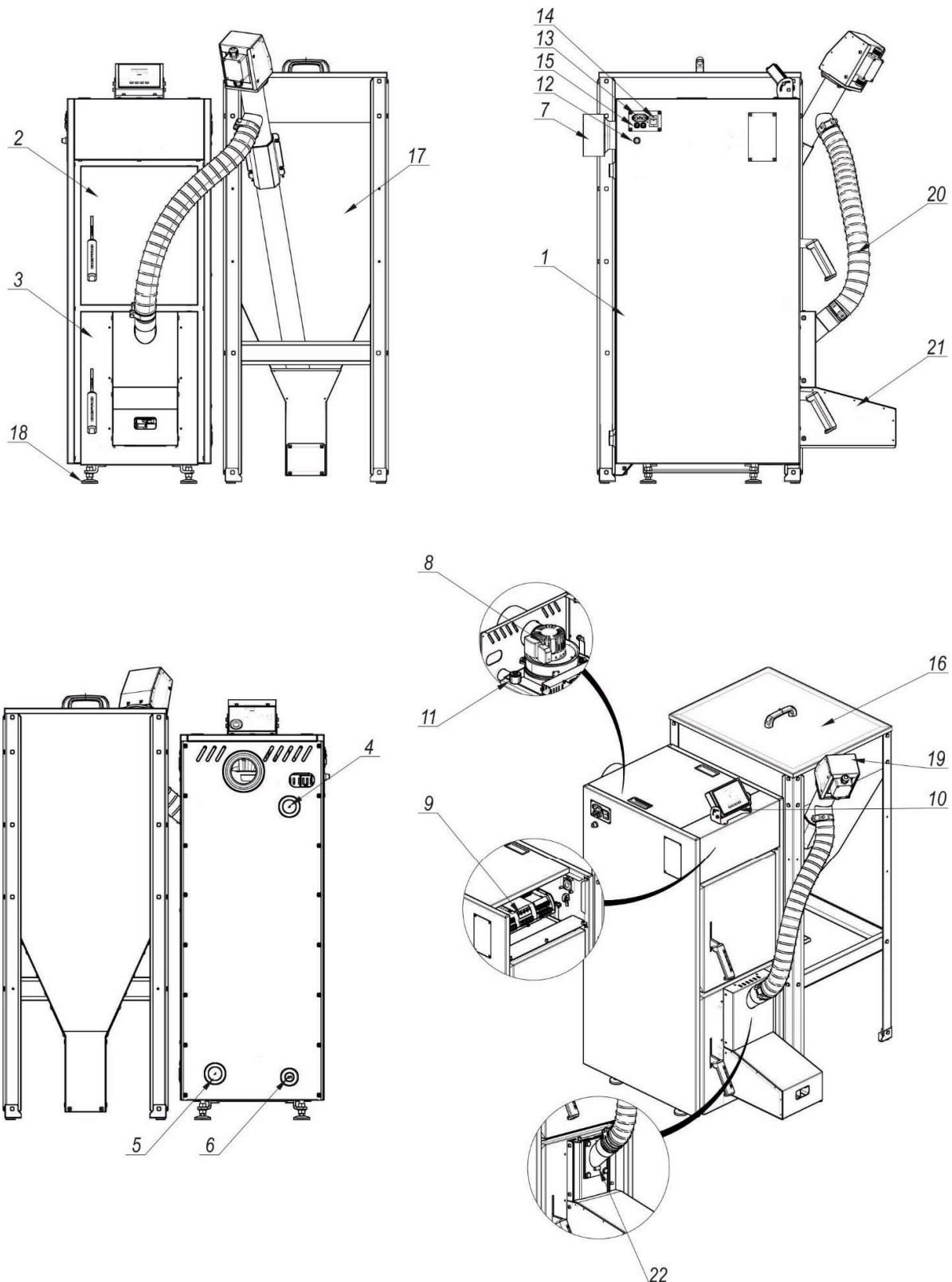
Abbildung 4. Kesselelemente NEXTPELL PLUS
