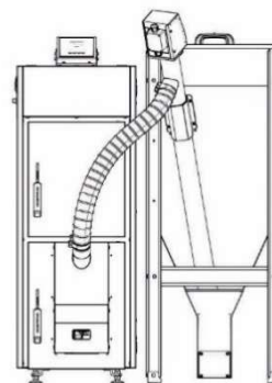
Abbildung 7. Position des Fallschlauchs
