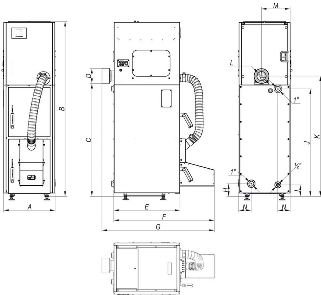
Abbildung 1. Abmessungen.
