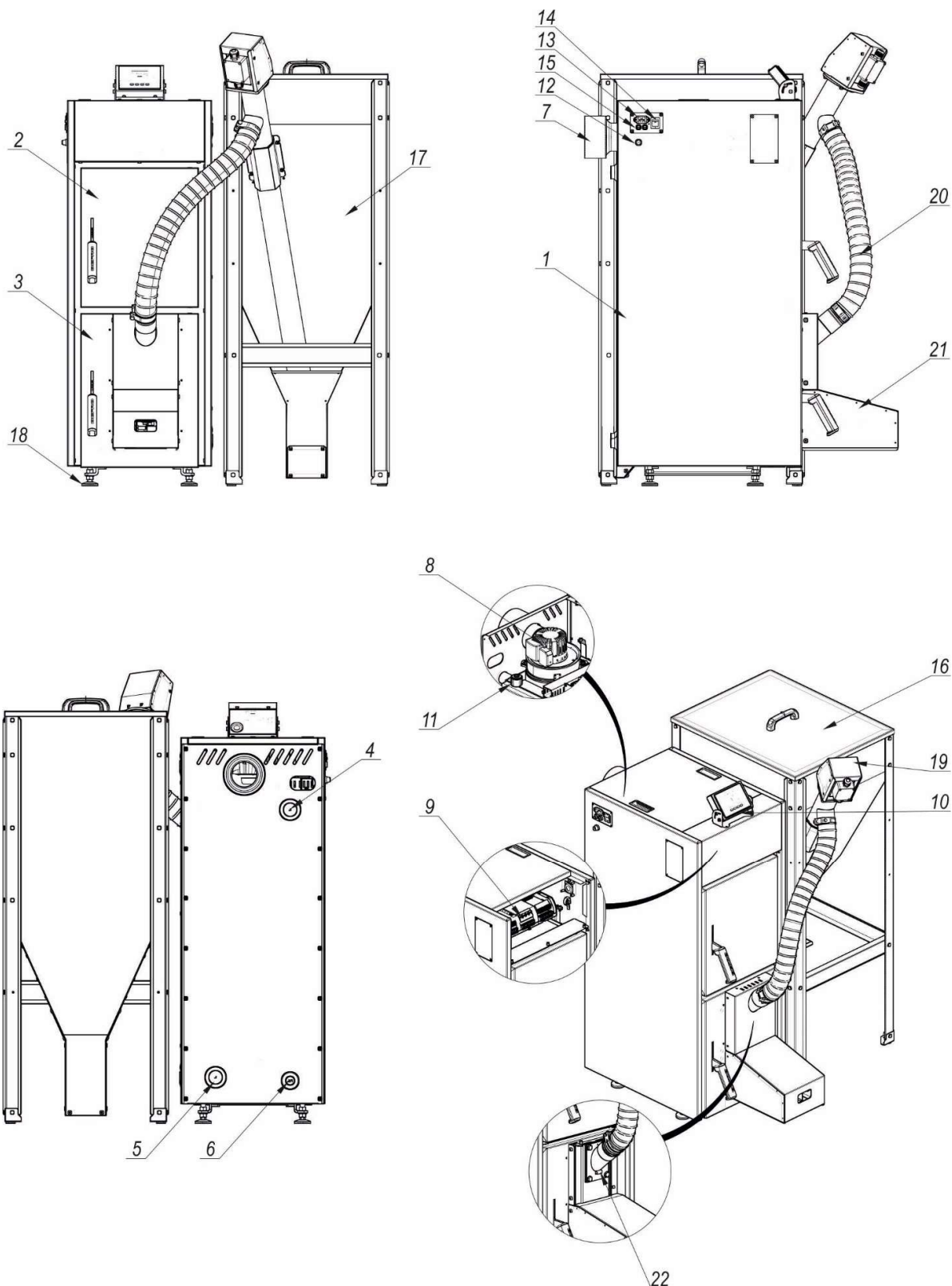
Abbildung 4. Kesselelemente NEXTPELL PLUS
